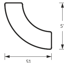
СЕЧЕНИЕ ПРОФИЛЯ
